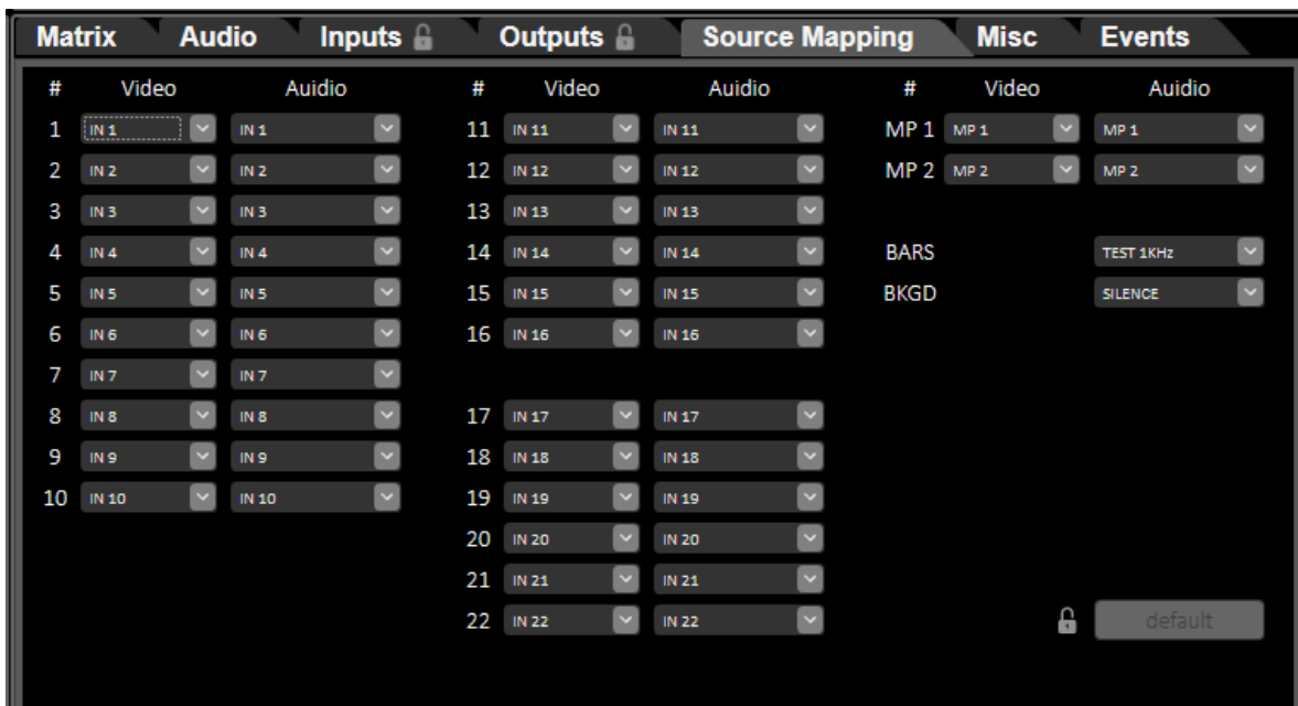
Рис. Закладка «Source Mapping» в программе «DSC10xx Switcher Control Panel», Конфигурация видео входов и внутренних источников микшера назначенных на кнопки пульта по умолчанию.
